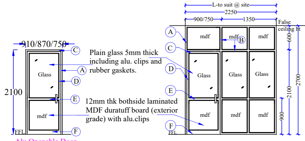
Alu. Openable Door D1 - 910 x 2100 Schedule item no: 39a D2 - 750 x 2100 Schedule item no: 39b D3 - 870 x 2100 Schedule item no: 39c
